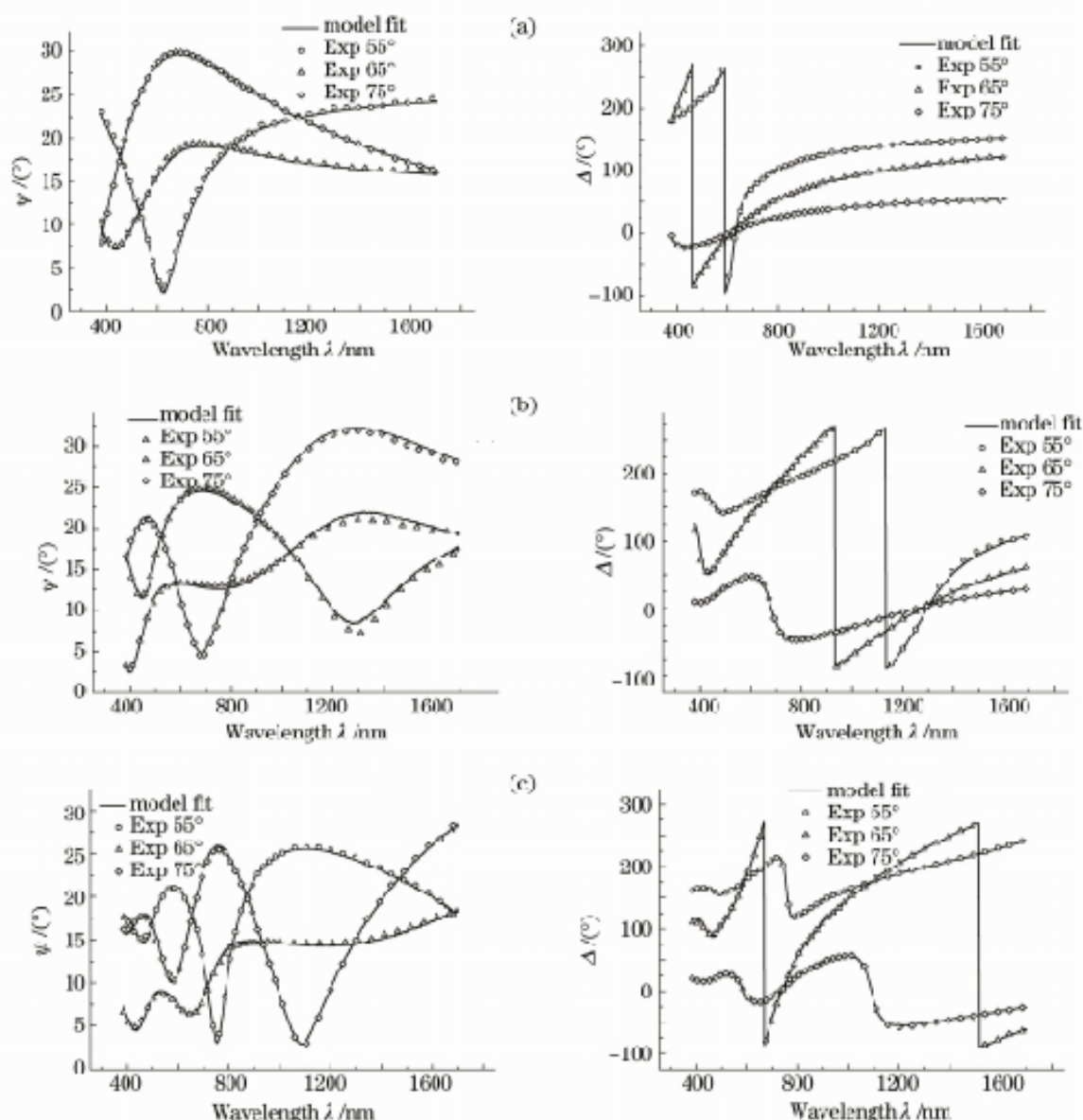
图 5 三个样品椭圆参数的模型计算值与实验值拟合情况。(a)1号样品;(b)2号样品;(c)3号样品
