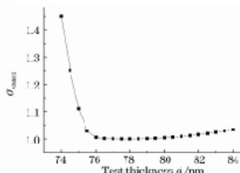
图2 单样品椭圆法实验厚度与 \sigma_{\text{MSE}} 关系
