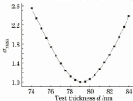
图 4 多样品分析法的实验厚度与 \sigma_{\text{NMSE}} 关系
