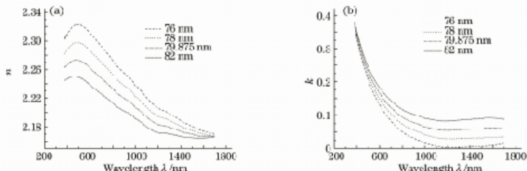
图3 样品在不同实验厚度下拟合得到的光学常数。(a)折射率,(b)消光系数
